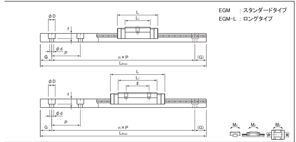
単位 : mm
