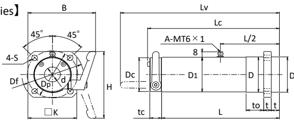
【LFWLB-MF-C series】
