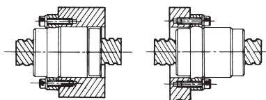
図67：ナット取付方法
