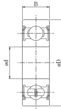
シールド形 ZZ
